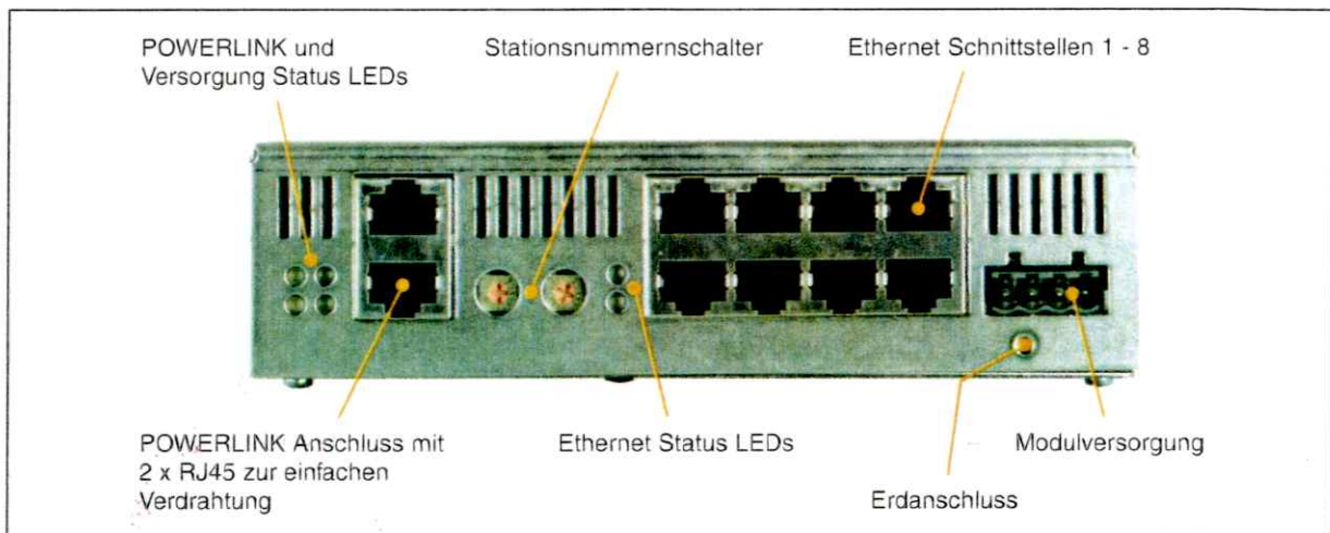
Abbildung 1: AK810 Bedien- und Anschlusselemente
